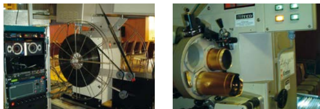
Projection classique de pellicule 35mm
